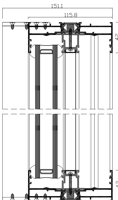
PRZEKRÓJ C-C
