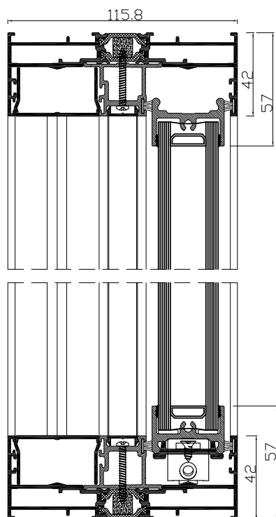
PRZEKRÓJ B-B
