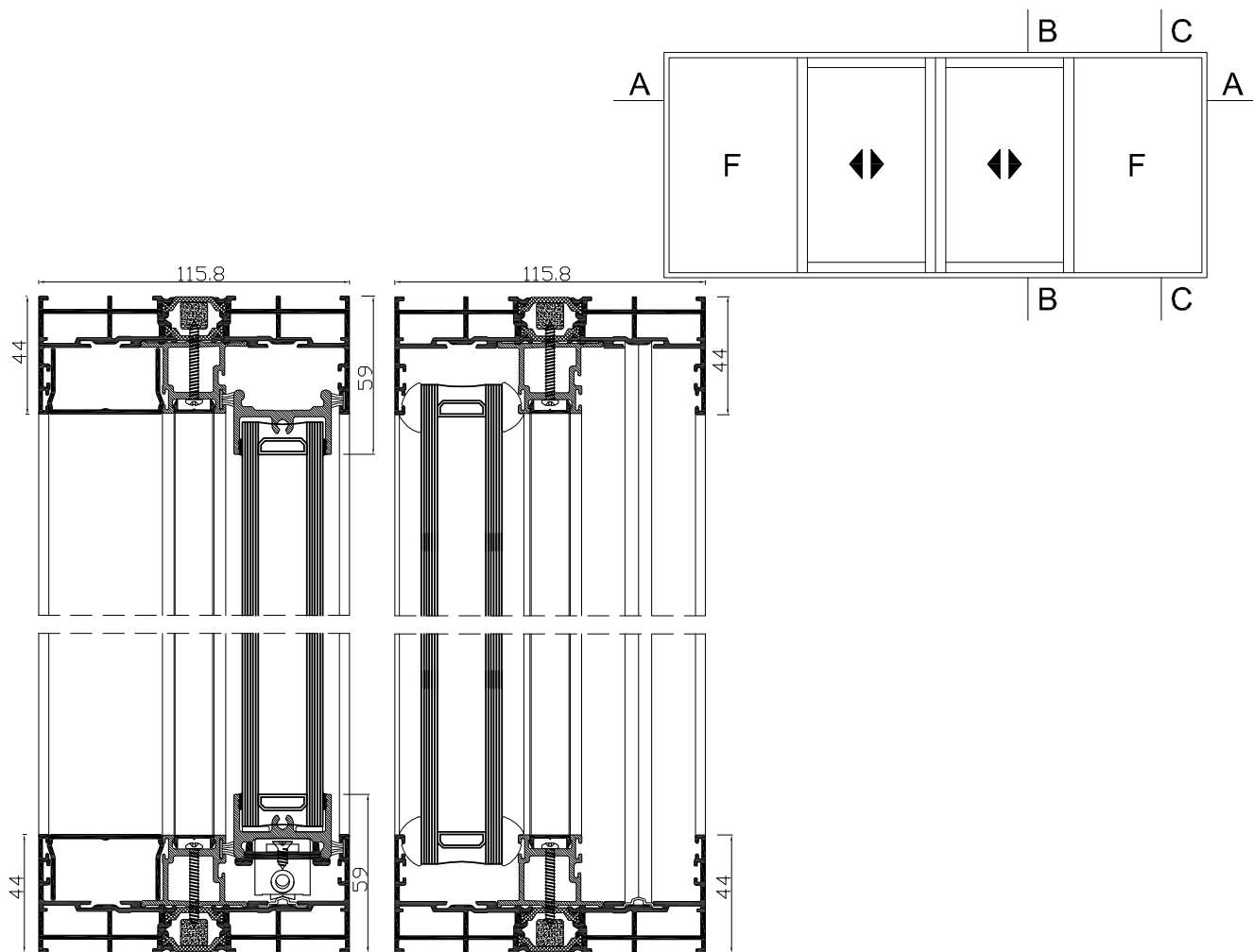
PRZEKRÓJ B-B
